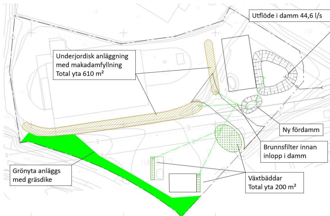
Figur 23. Föreslagen dagvattenhantering inom planområdet. Infarten flyttad enligt Figur 15. (Dagvattenutredningen)
