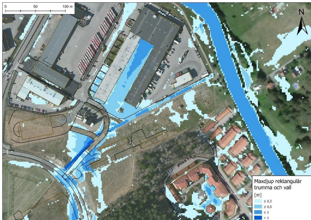
Figur 20. Visar maxdjup med en rektangulär trumma under den nya planerade infarten till Säbydepån. Infarten till planområdet flyttas därför enligt Figur 15. Pilar visar de större rinnvägarna från uppströms områden. (Dagvattenutredningen)
