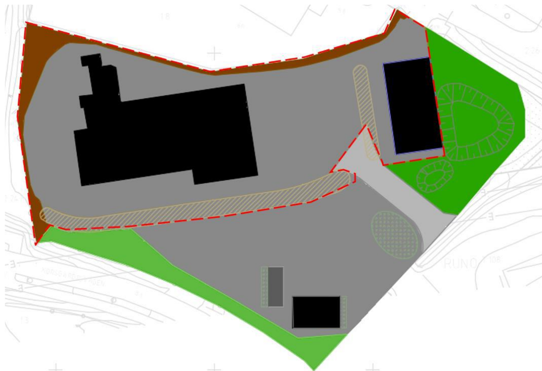
Figur 25. Ytor som avleds till makadammagasin är inringade med röd streckad linje. Infarten flyttad enligt Figur 15. (Dagvattenutredningen)
