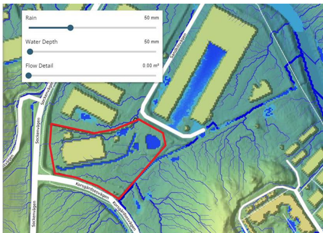
Figur 17. Områden med risk för översvämning med vattendjup mer än 50 mm i befintlig situation är markerade med blått. Plangränsen är markerad med röd linje. (Dagvattenutredningen)
