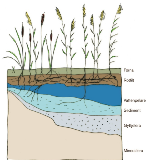
Figur 34 De olika lagren i ett vassbälte ovanifrån: Förna, Rotfilt, Vattenpelare, Sediment, Gyttjeleran och Minerallera. Illustrationen är inspirerad av förstudien "Askövikens, Förutsättningar för en Blå bärd" (efter Jobansson, 2002) samt från Askövikens "blå bärd" (Jobansson & Rehnberg, 2008). Principen är den samma vid Täljöviken. IllustrationMen : Ekologigruppen .
