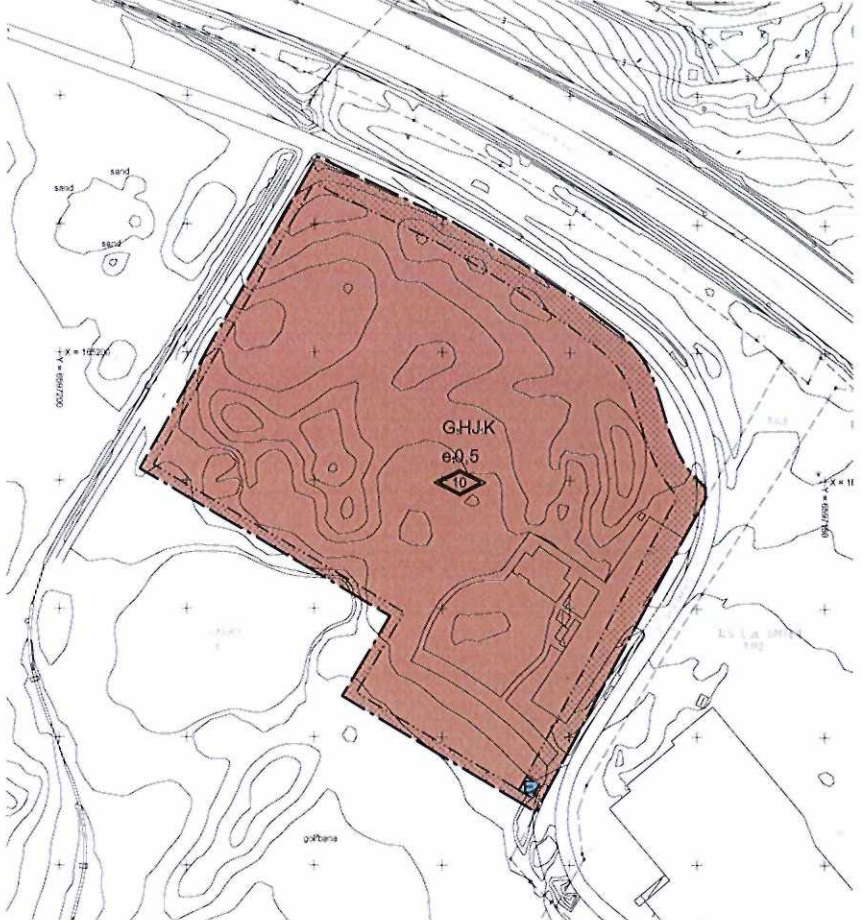
PLANKARTA
