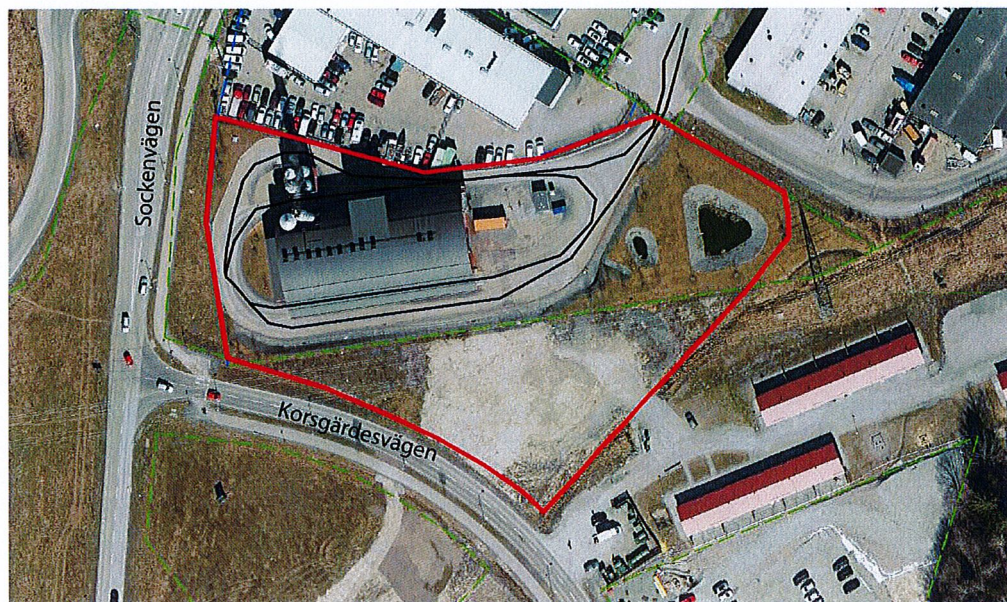
Figur 14. Befintligt vägnät inom och intill planområdet. Plangränsen ses som röd linje medan viktiga körvägar inom planområdet visas som svarta linjer.
