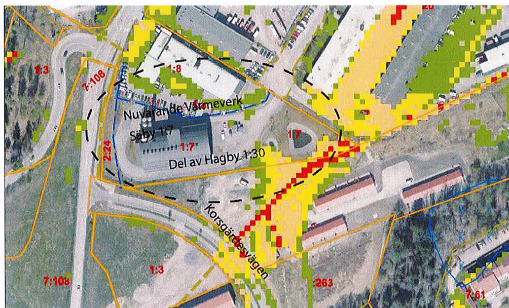
Figur 19. Resultat av översvämningsanalys med Mike 21. (Dagvattenutredningen)
