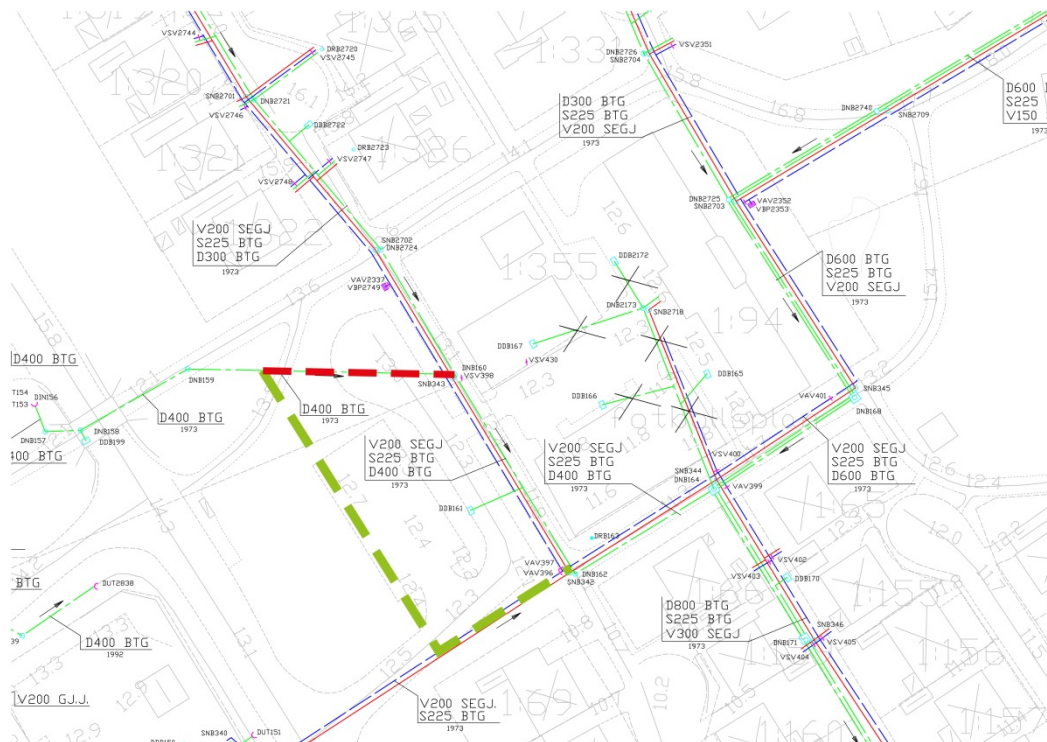
Bild 17. Förslag på ny dragning av dagvattenledning markeras med streckad linje i grönt, befintlig ledning visas i rött.
