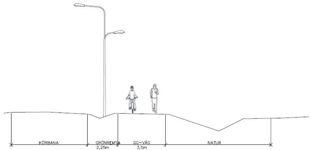
Figur 2. Gång- och cykelväg med 2,25 meter skiljeremsa. Illustration: Ramböll och Sara Hägg
