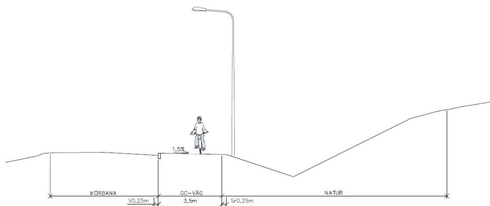
Figur 4. Gång- och cykelväg med kantsten. Illustration: Ramböll och Sara Hägg
