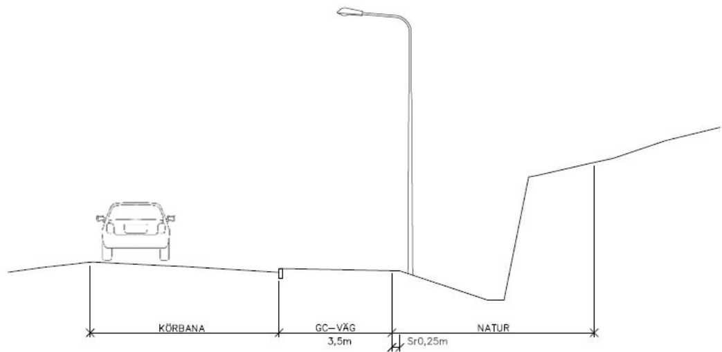
Figur 3. Gång- och cykelväg med kantsten och bergskärning. Illustration: Ramböll och Sara Hägg
