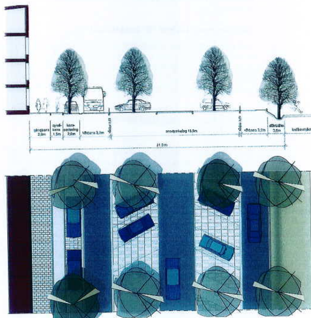
Esplanaden (södra huvudgatan) 31 m
